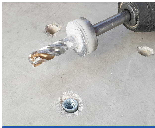
Zum Setzen von Einschlagankern
