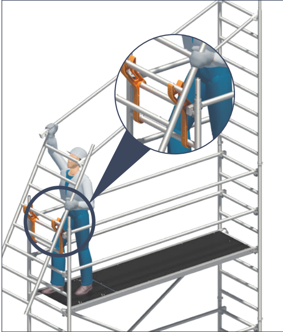
1 Aufstecken der ersten Standleiter. Anbringen der Uni Montagehaken und Positionierung der zweiten Standleiter zur Montage der Geländer.
