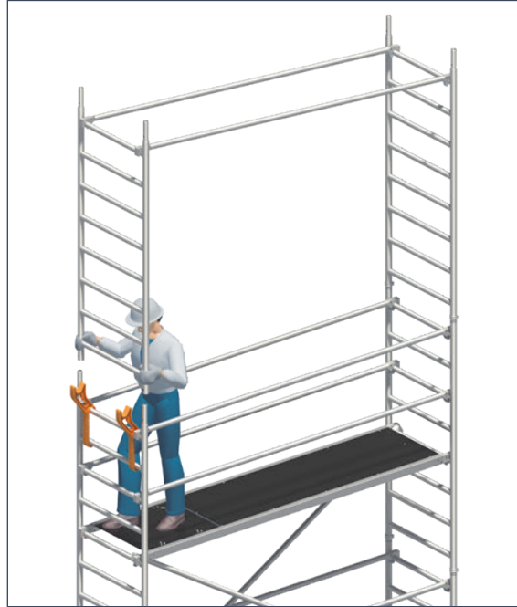
2 Standleiter mit Geländer nach oben schwenken und aufstecken.
