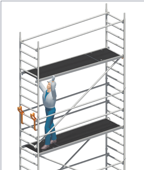
3 Diagonalen und Durchstiegsbrücke einsetzen.
