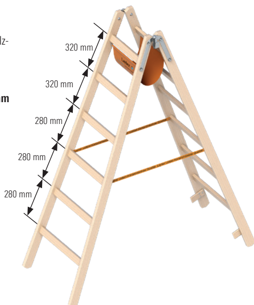
Holzstehleiter 1053 nach Ö-Norm Z1501
